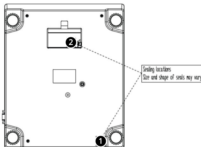
Fig. 2 : Emplacement des marques de scellement
